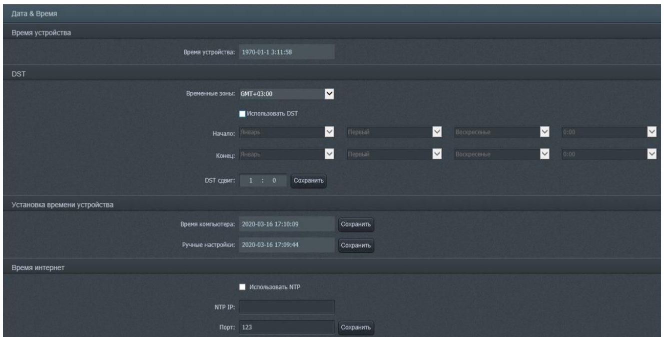
Рисунок 10 - Подменю «Время»
