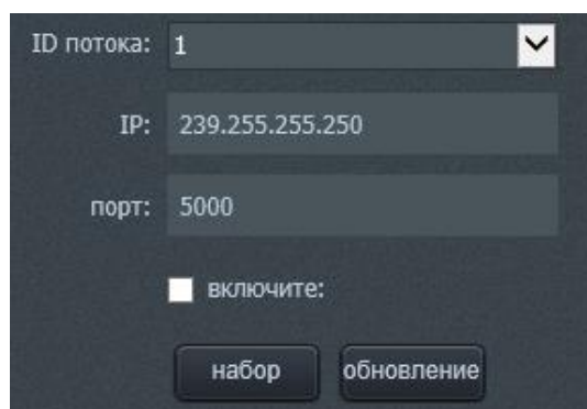
Рисунок 32 – Подменю «RTP»
