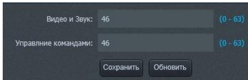
Рисунок 11 - Вкладка «QoS»
