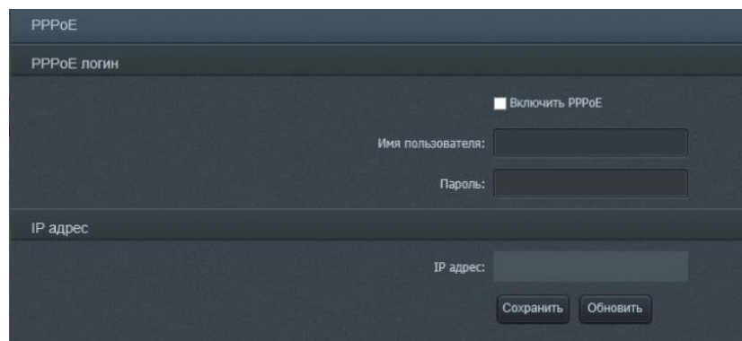
Рисунок 8 – Подменю «PPPoE»
