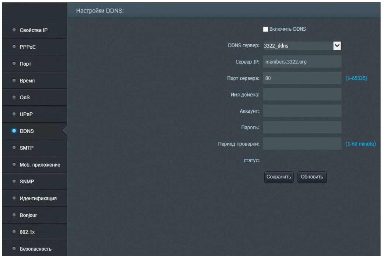
Рисунок 13 – Подменю «DDNS»
