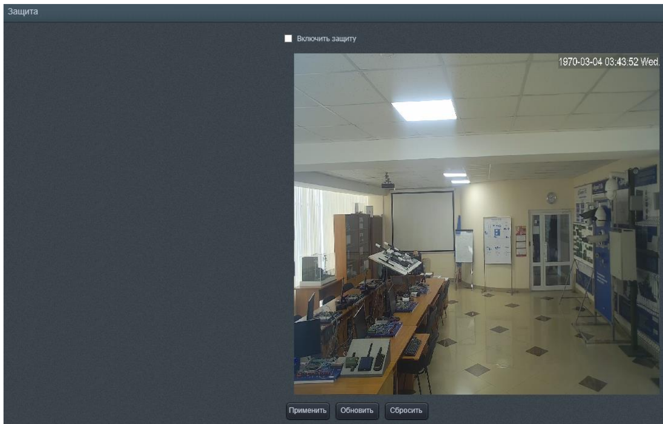
Рисунок 27 – Подменю «Защита»
