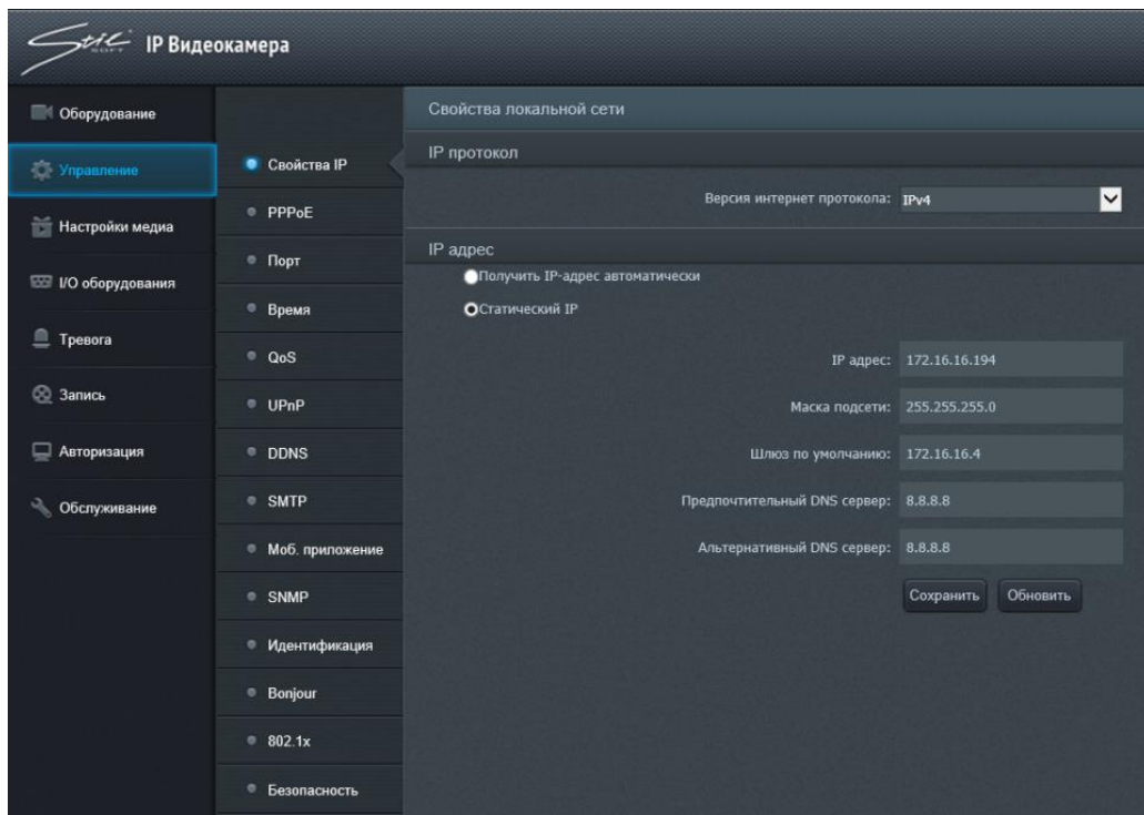
Рисунок 7 – Меню «Управление»
