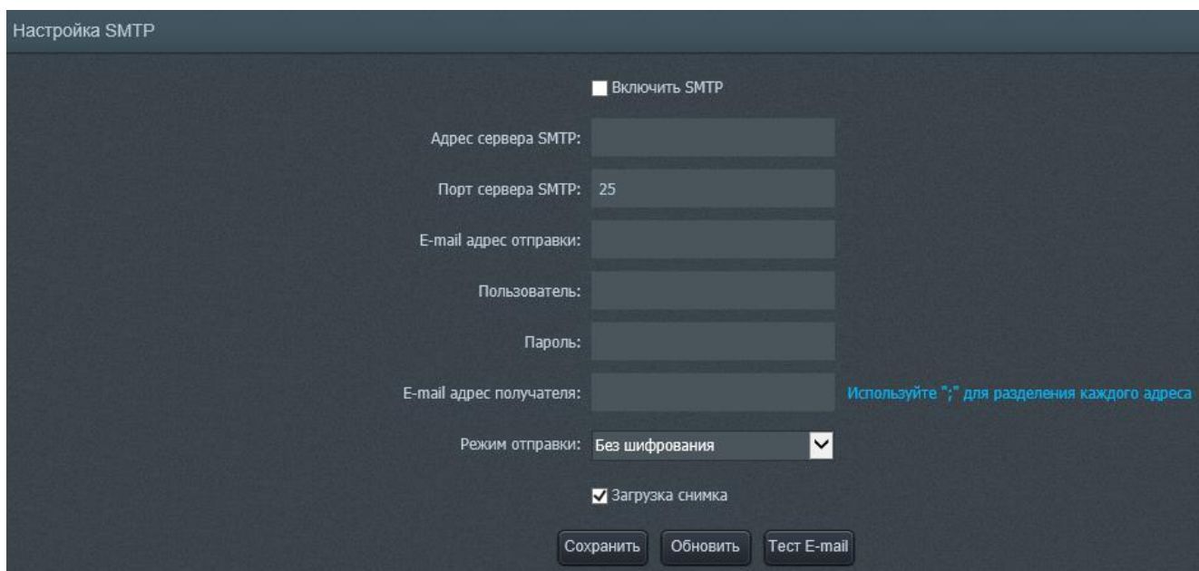
Рисунок 15 – Настройка «SMTP»
