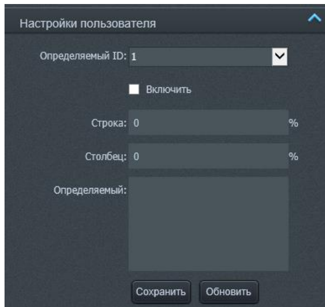
Рисунок 26 – Подменю «OSD»
