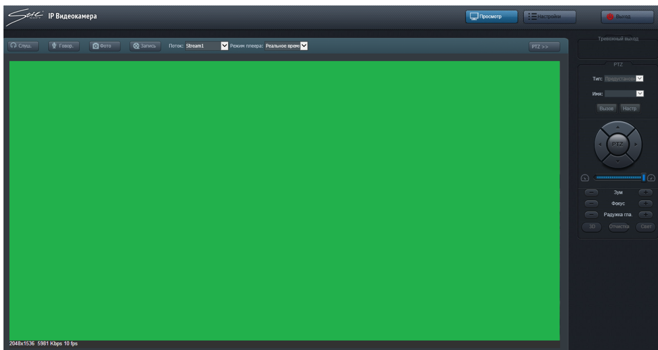
Рисунок 5 – Окно видеоканала
