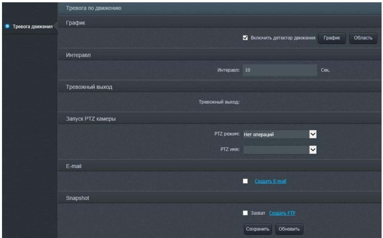
Рисунок 35 – Вкладка «Тревога»
