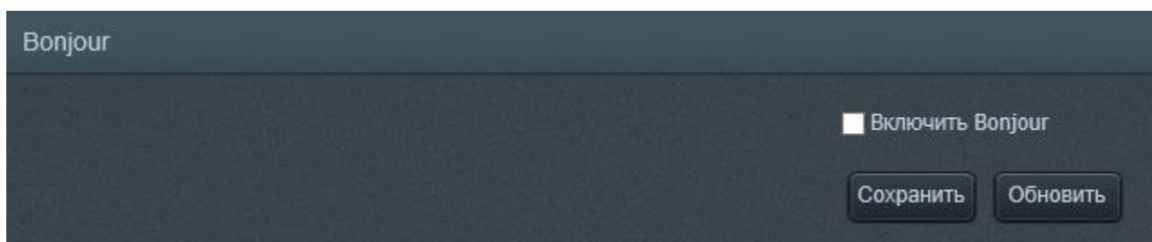
Рисунок 20 - Подменю «Bonjour»
