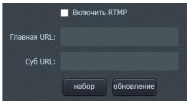
Рисунок 32 – Подменю «RTMP»
