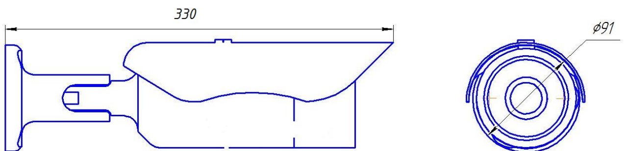
Рисунок 2 – Габаритные размеры IP-видеокамеры SDP-858I
