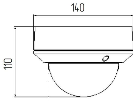
Рисунок 2 – Габаритные размеры изделия SDP-855
