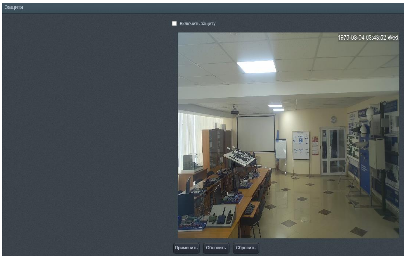
Рисунок 28 – Подменю «Защита»
