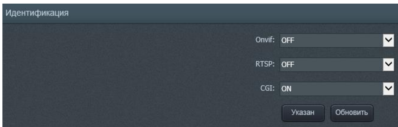
Рисунок 19 - Подменю «Идентификация»
