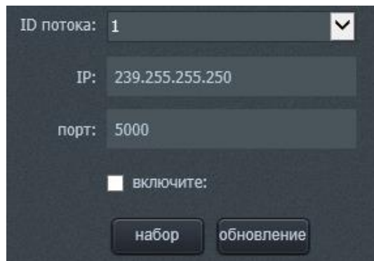
Рисунок 32 – Подменю «RTP»
