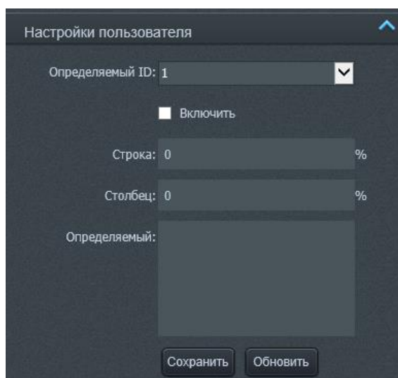
Рисунок 27 – Подменю «OSD»
