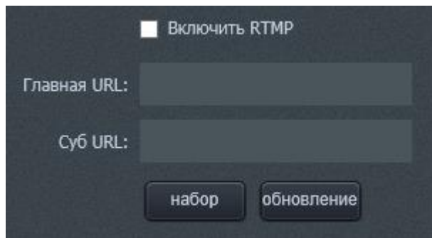
Рисунок 31 – Подменю «RTMP»
