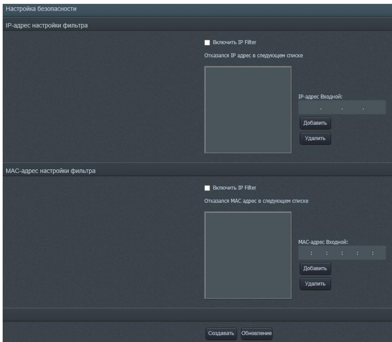
Рисунок 22 - Подменю «Безопасность»
