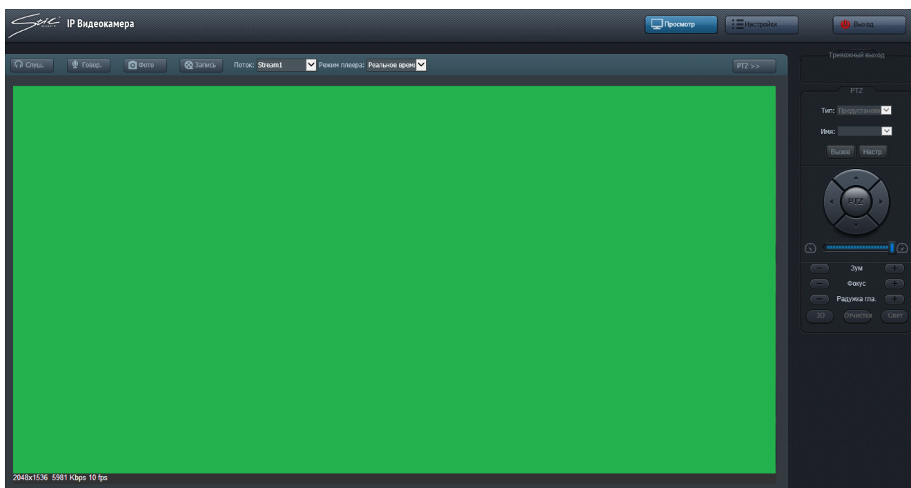
Рисунок 7 – Окно видеоканала
