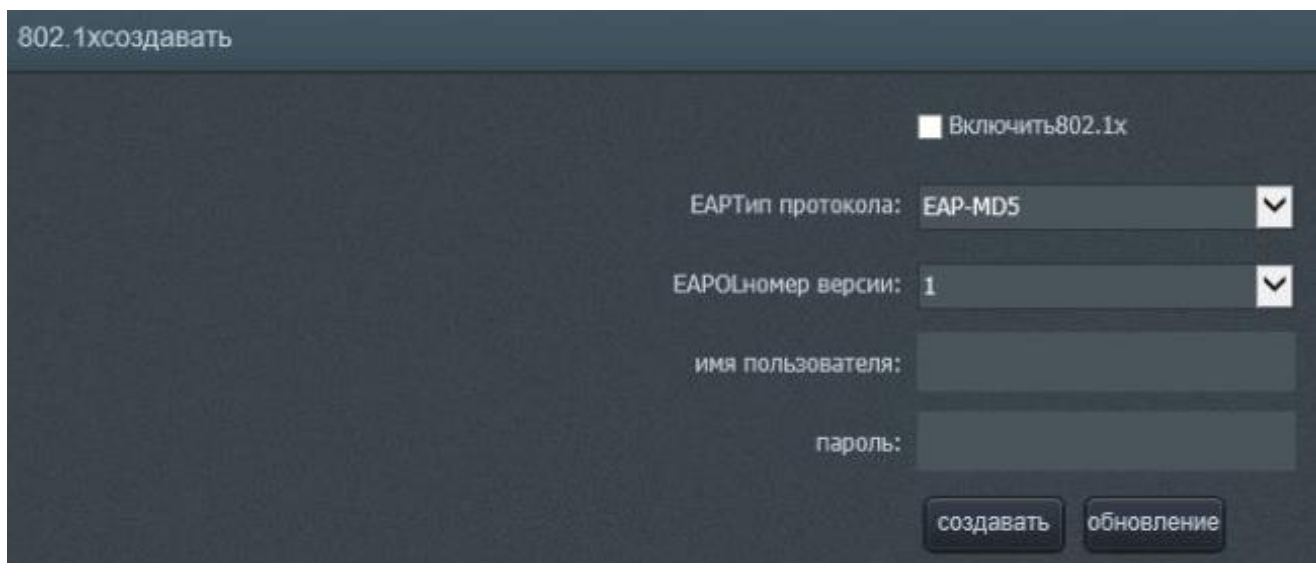
Рисунок 21 - Подменю «802.1x»
