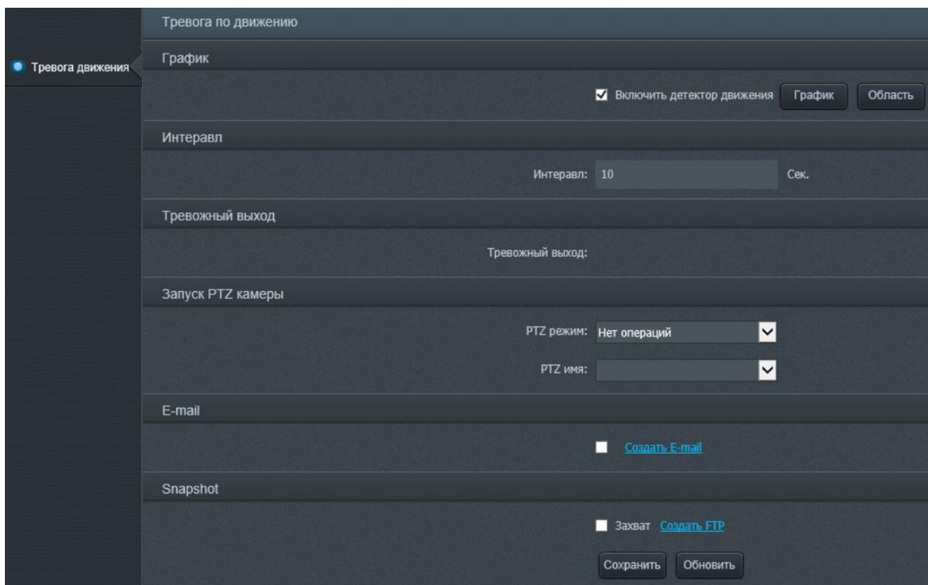
Рисунок 34 – Вкладка «Тревога»
