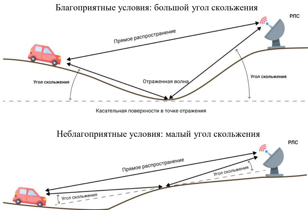
Рисунок 5. Зависимость обнаружения от угла скольжения.
