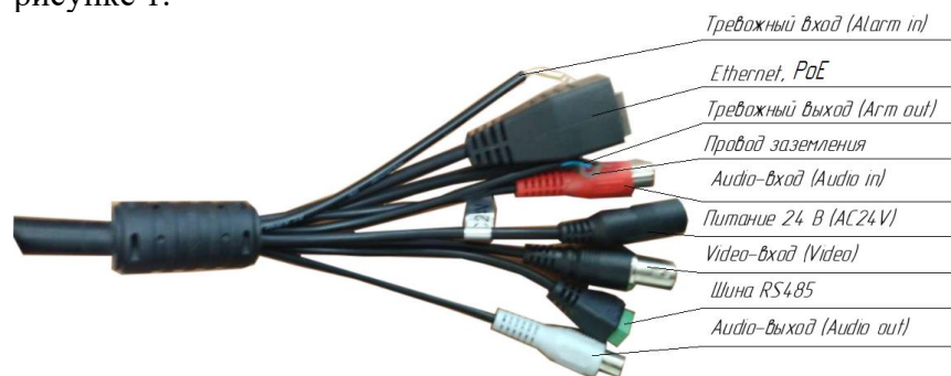
Рисунок 1 – Подключение IP-видеокамеры
