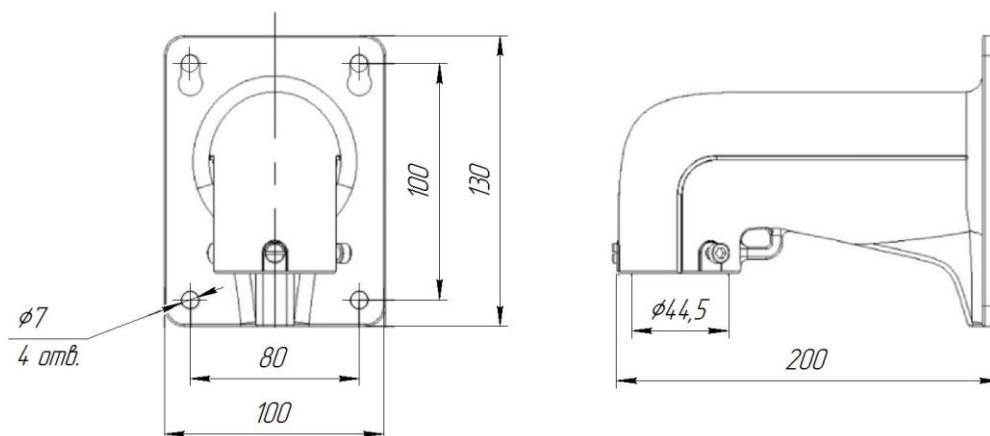
Рисунок 3 – Габаритные размеры кронштейна IP-видеокамеры SDP-850
