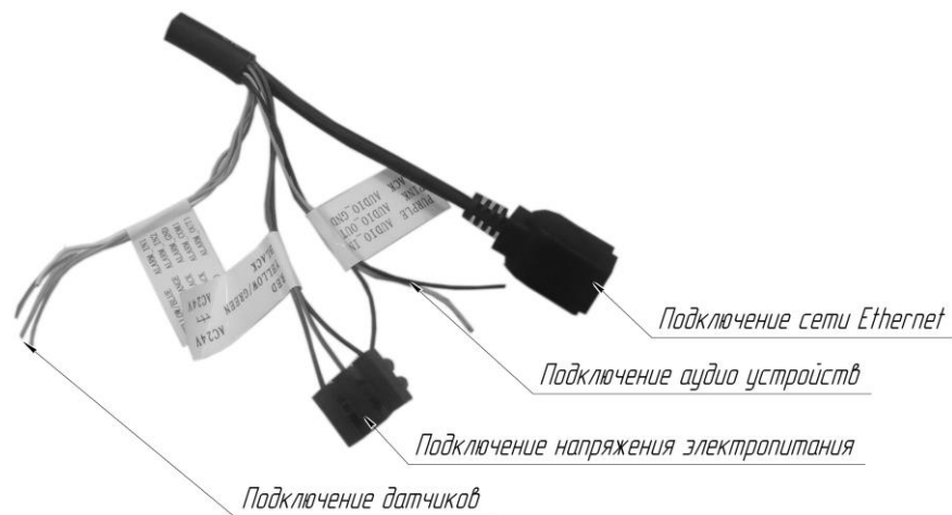
Рисунок 4 – Кабели подключения IP-видеокамеры SDP-850
