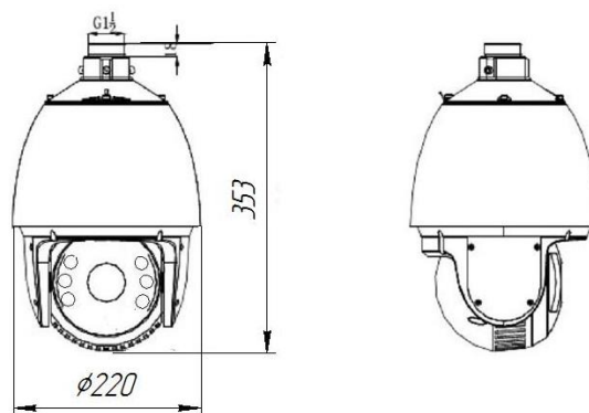
Рисунок 2 – Габаритные размеры IP-видеокамеры SDP-850
