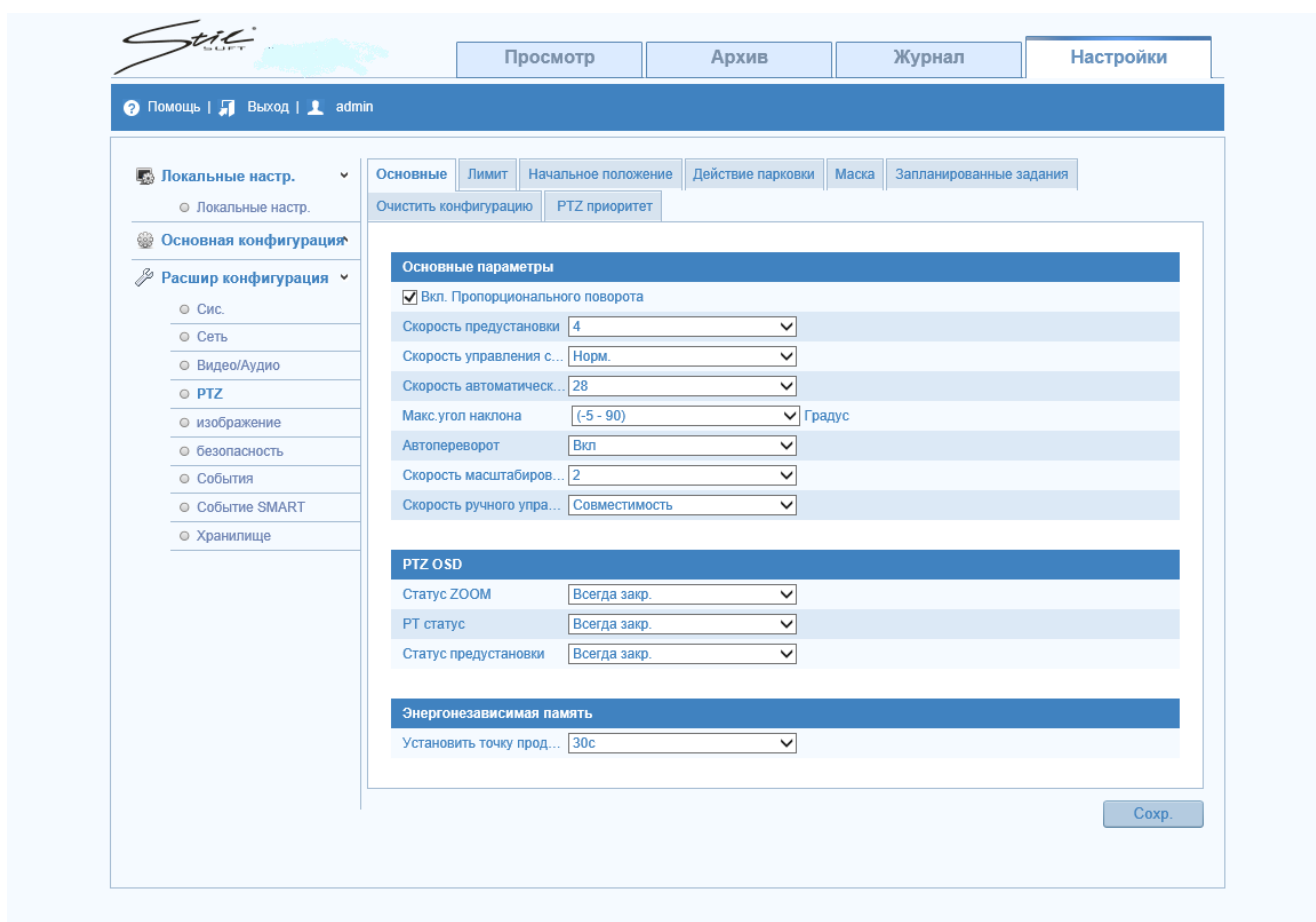
Рисунок 15 – Окно настроек поворотного устройства
