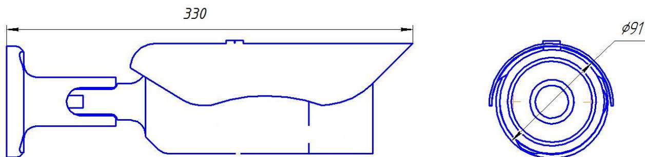
Рисунок 2 – Габаритные размеры видеокамеры СВК-858И
