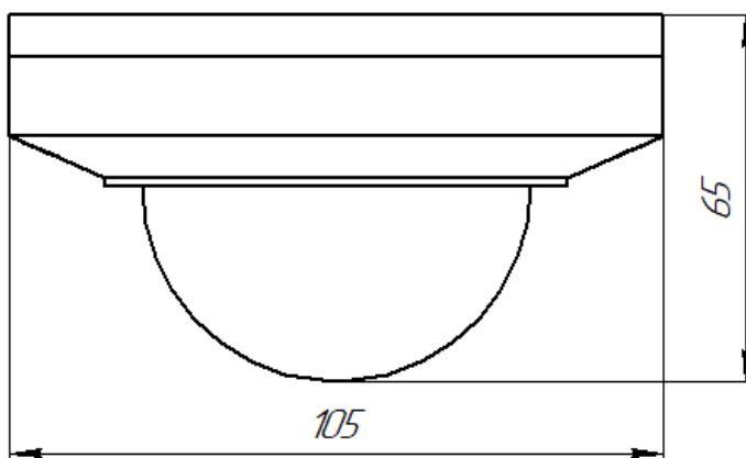
Рисунок 2 – Габаритные размеры видеокамеры СВК-859
