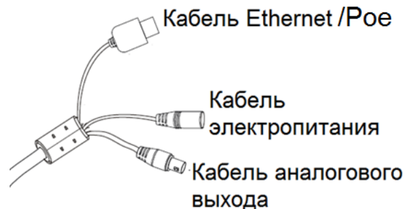
Рисунок 1 – Подключение IP-видеокамеры
