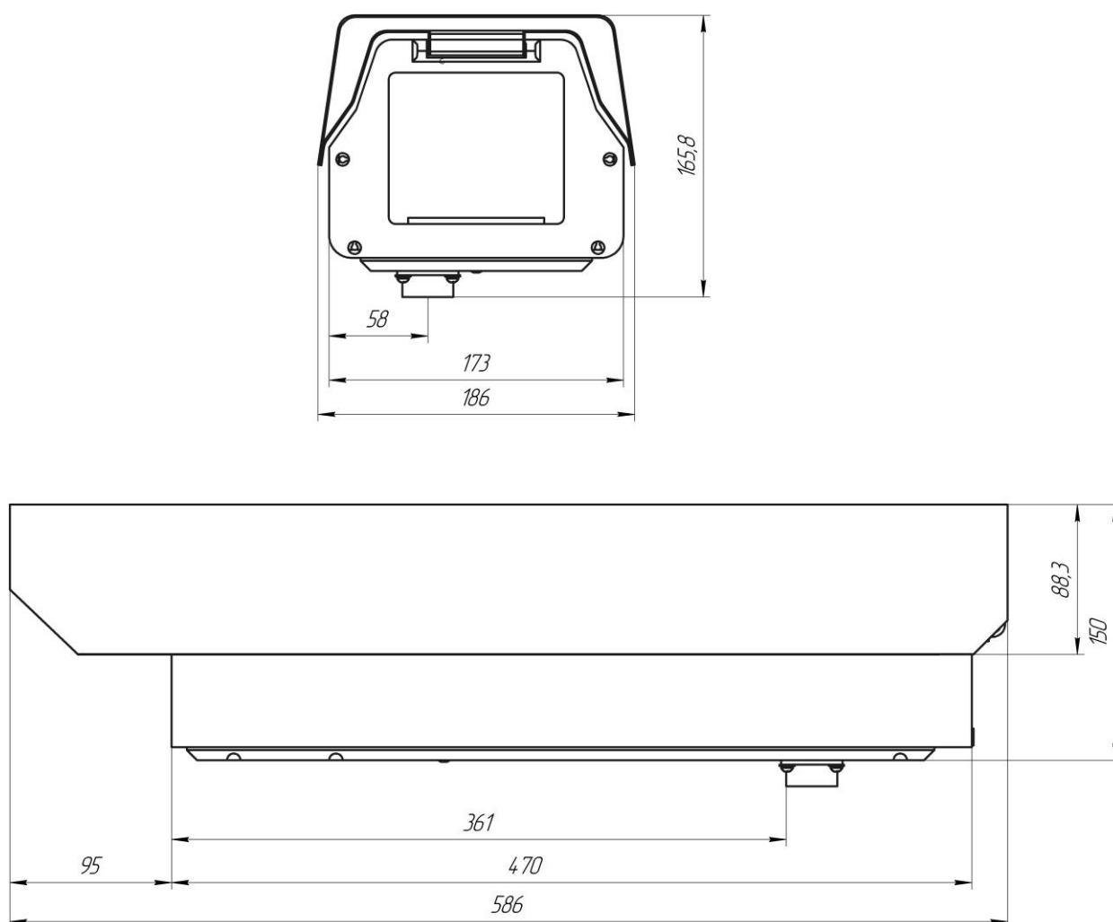
Рисунок 2 – Габаритные размеры видеокамеры TBS-USD
