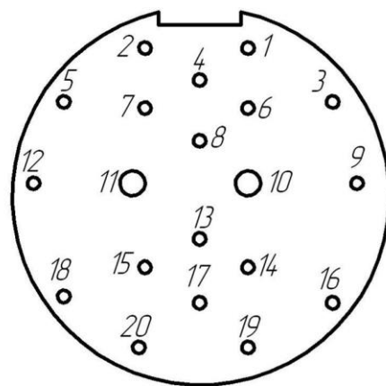
Рисунок 1 – Обозначение контактов разъема (вилки) подключения тепловизора
