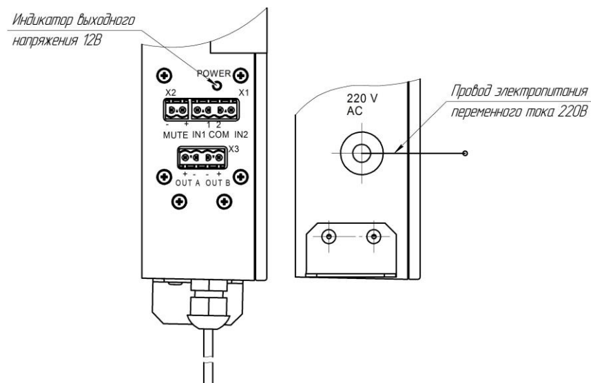
Рисунок 1 – Подключение трансляционного аудиоусилителя
