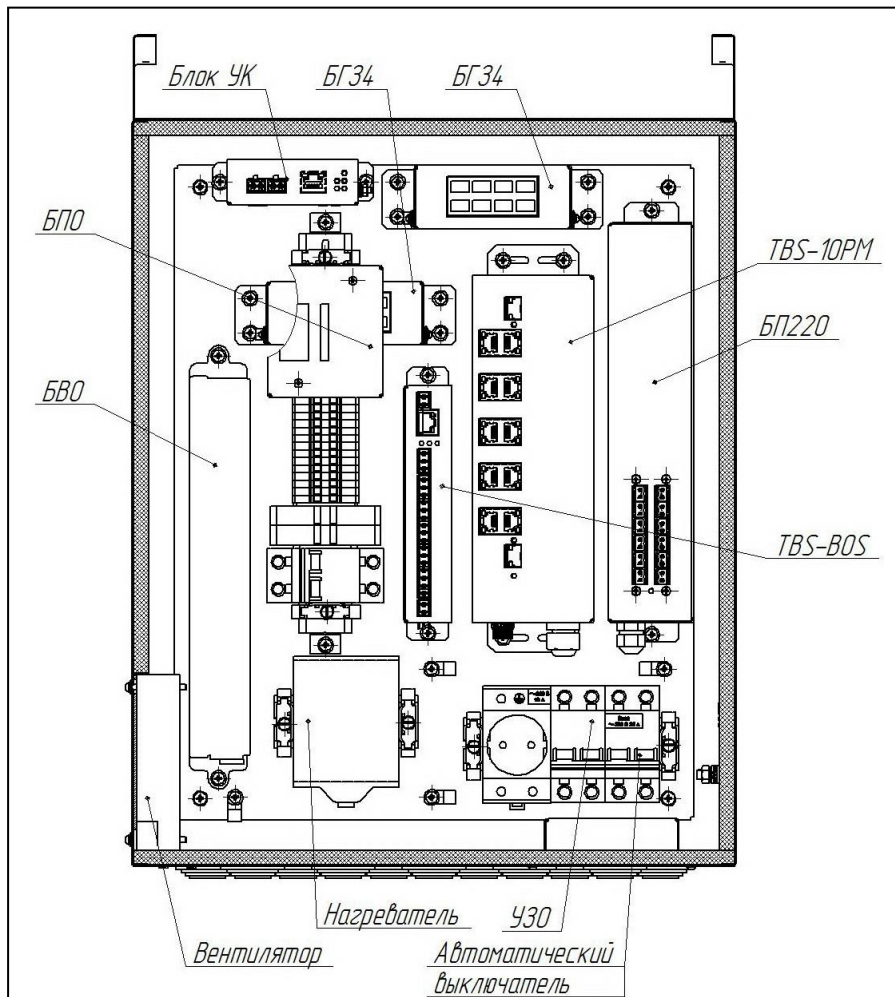
Рисунок 1 – Размещение блоков на монтажной панели
