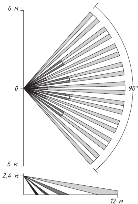
Рисунок 3 – Конфигурация зоны обнаружения извещателя
