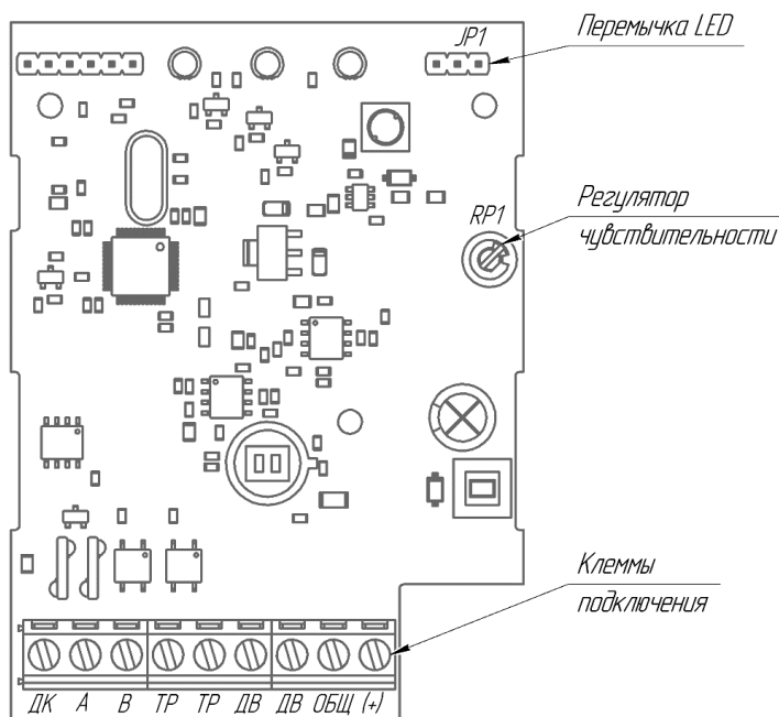
Рисунок 2 – Плата с разъёмами подключения и регуляторами чувствительности
