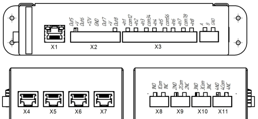
Рисунок 1 – Назначение разъемов контроллера
