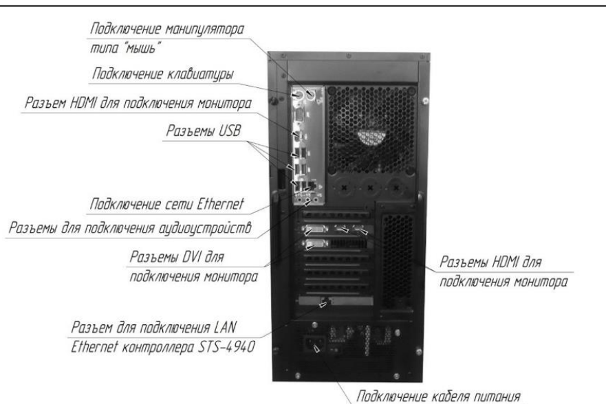
Рисунок 1 – Подключение сервера (расположение, внешний вид, типы разъемов и их количество может отличаться от приведенного)
