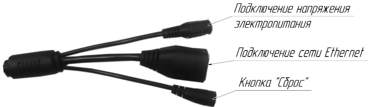
Рисунок 3 – Кабели подключения видеокамеры SDP-858I
